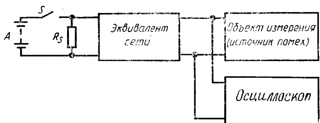
Схема измерения напряжения помех
