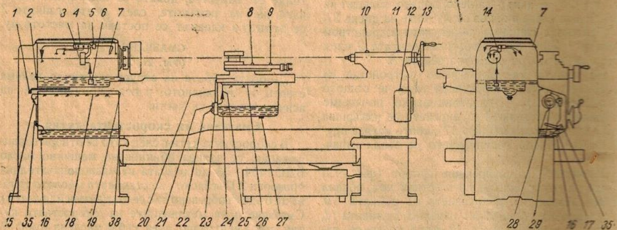
Фиг. 27. Схема на смазването
