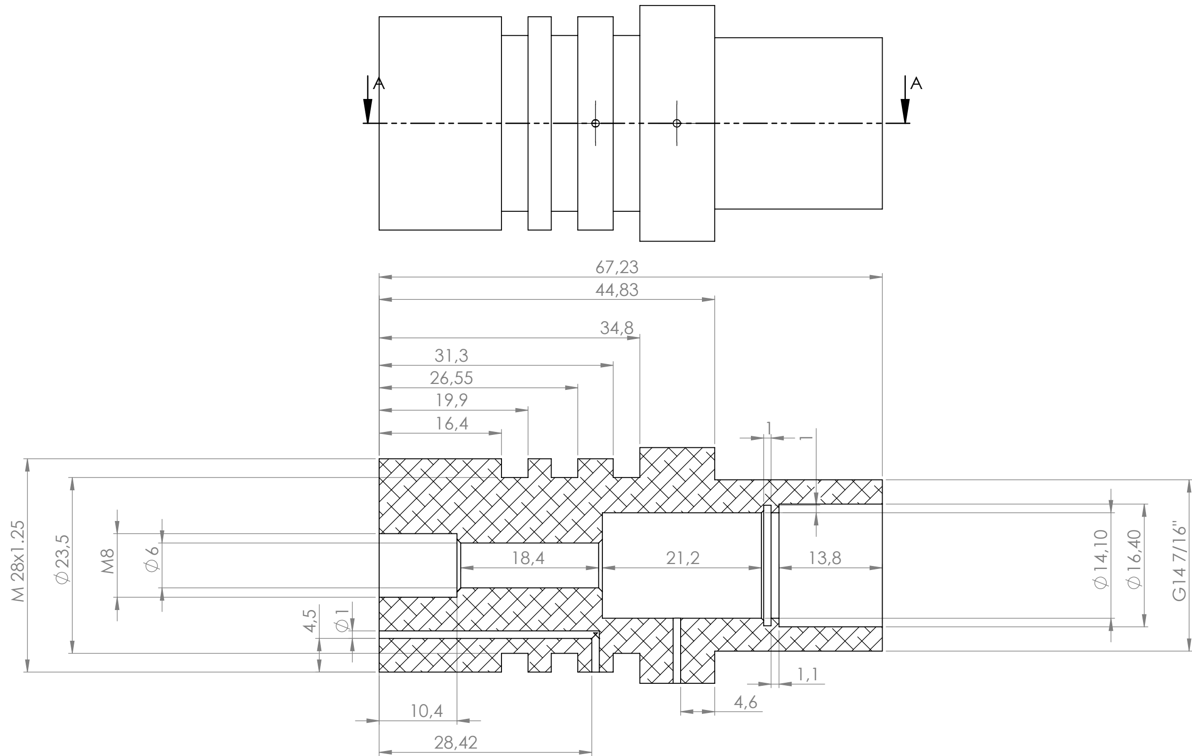
SECTION A-A
