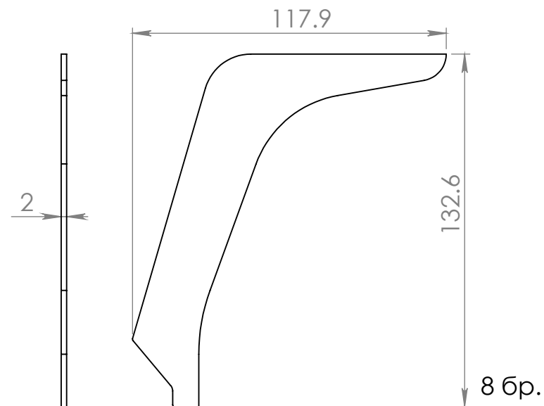
Държач релинг страница -3mm
