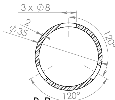
B-B 1 : 1
