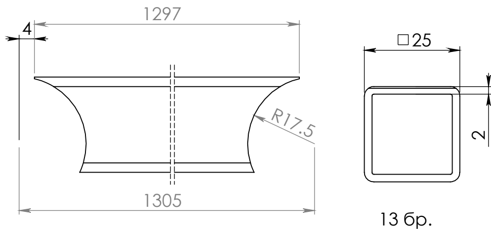
Напречно долен релинг
