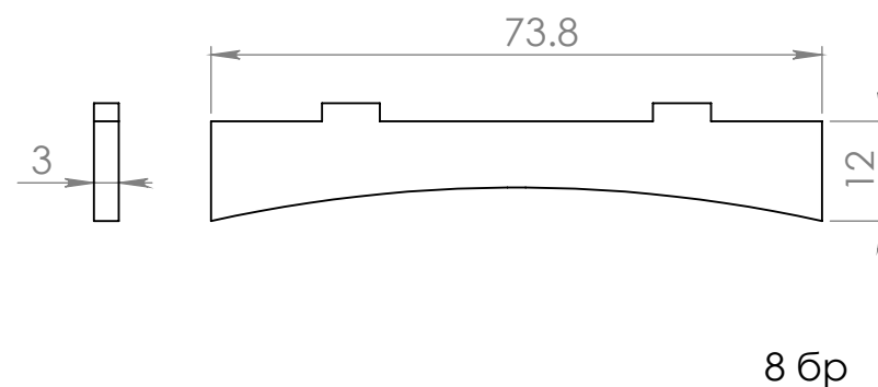
Държач релинг ребро 02
