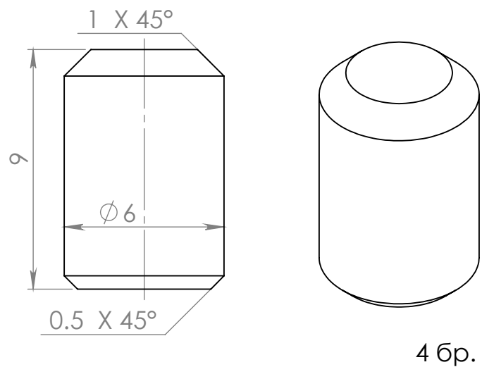
щифт 10x \phi 6 mm
