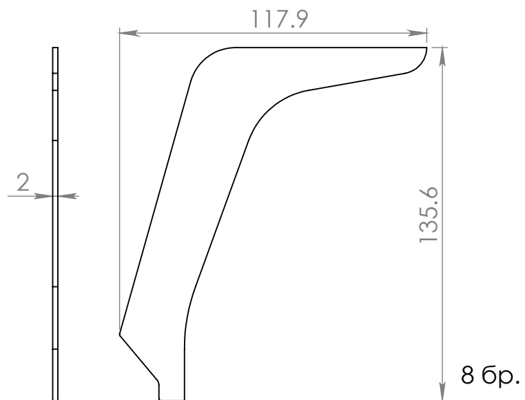
Държач релинг страница
