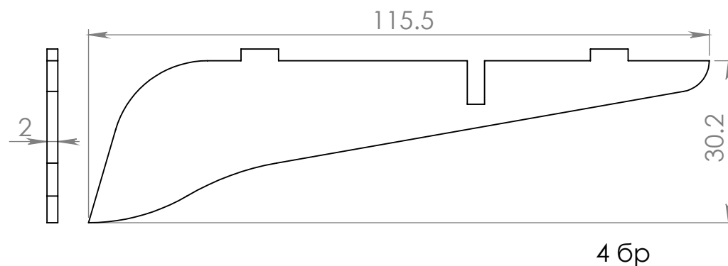
Държач релинг ребро 01 -3mm
