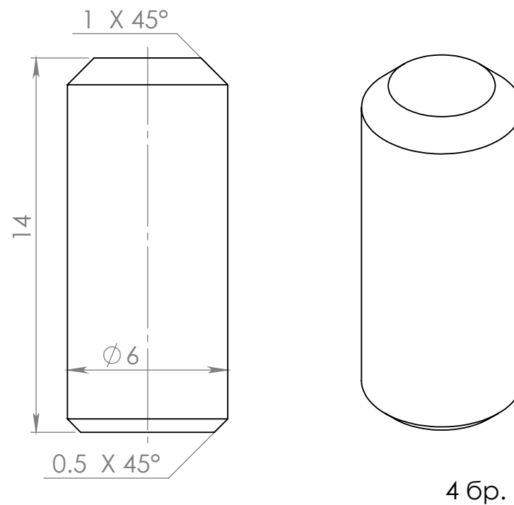
щифт 15x \phi 6 mm
