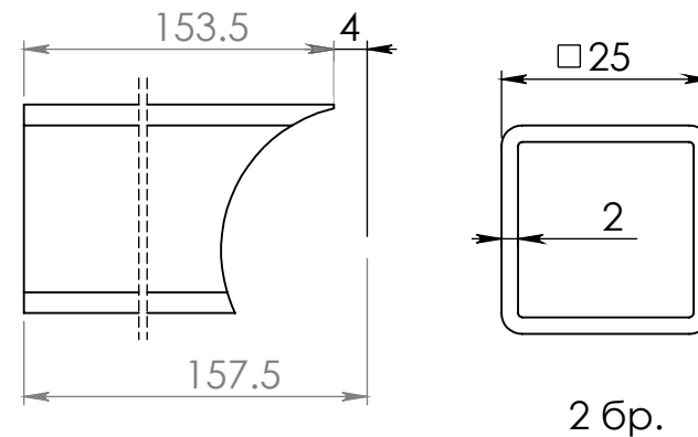
Напречно отзад долен релинг
