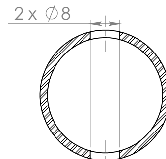
E-E 1 : 1
