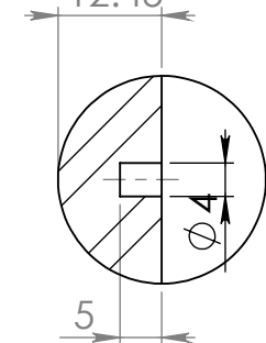
SECTION D-D
